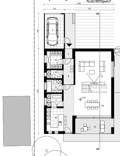
Hiša 2: tloris pritličja
