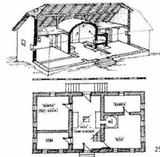
25: osrednjeslovenska hiša, Stara vas na Bizeljskem (vir: Fister, 1993)
