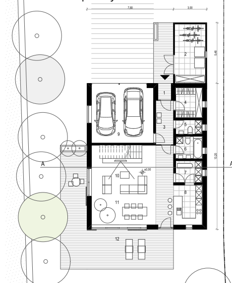
Hiša 1: tloris pritličja
