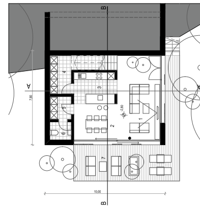
tloris pritličja
