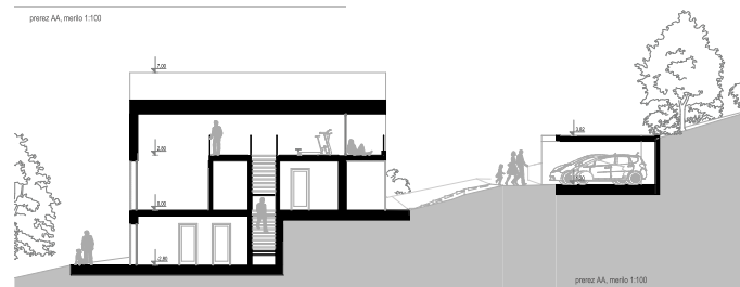
Prerez stanovanjske hiše
