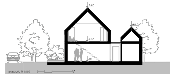
Prerez
