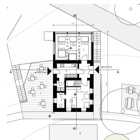
Tloris pritličja
