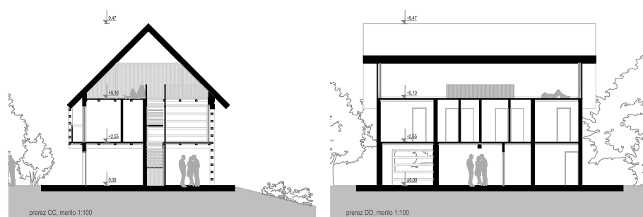
Prerez gospodarskega objekta
