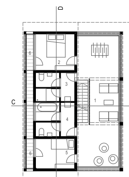
Tloris nadstropja
