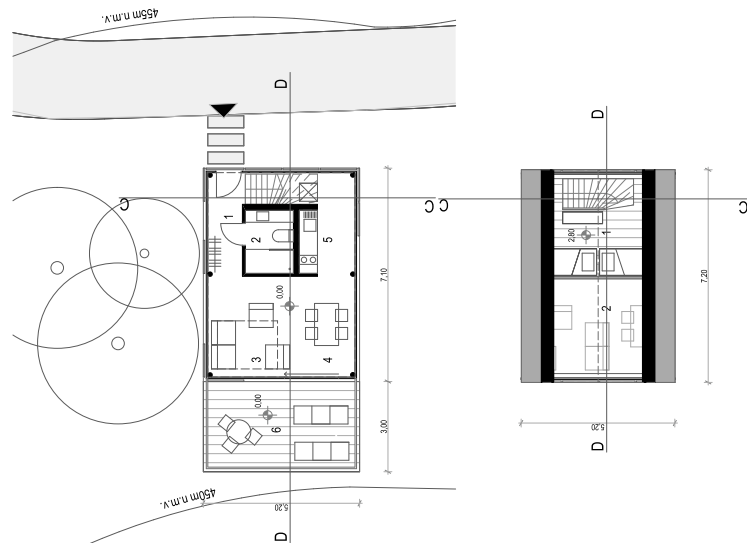
Turistični apartma: tloris pritličja tloris nadstropja
