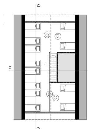
Tloris mansarde
