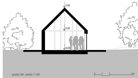
Prerez hiše
