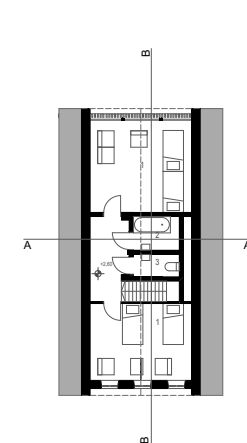
Tloris mansarde
