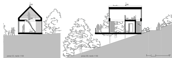
Prerezi: turistični apartma
